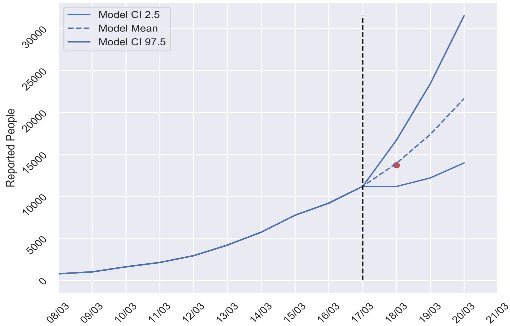
Figura 2: Predicción de reportados respecto al COVID-19 en ESPAÑA entre entre los días 17/03/2020 y 20/03/2020. Los puntos rojos corresponden a los datos publicados posteriormente a la realización de esta predicción. IMPORTANTE LEER APARTADO ACTUALIZACIÓN INFORME.
