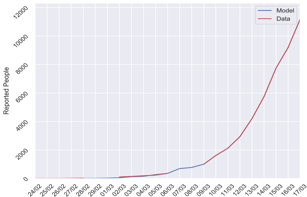
Figura 1: Reportados con COVID-19 en ESPAÑA entre entre los días 24/02/2020 y 17/03/2020. La línea roja corresponde a los datos de reportados por COVID-19. La ausencia de datos reportados
