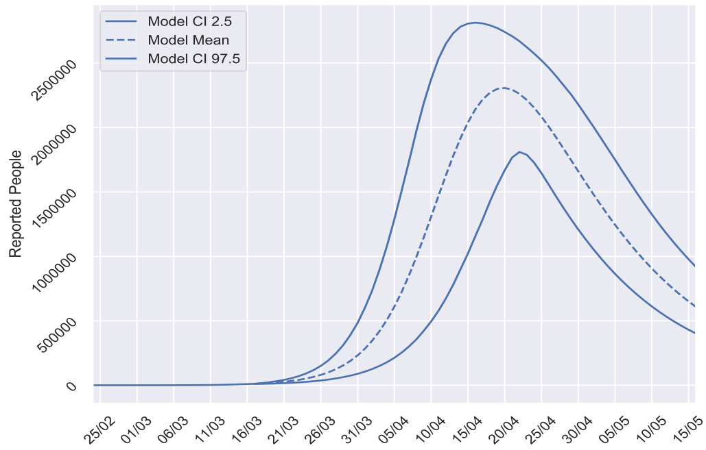
Figura 3: Predicció a largo plazo de la evolución del número de casos reportados de COVID-19.
