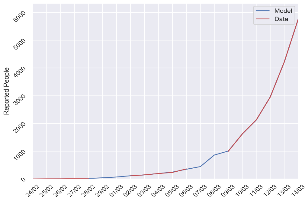
Figura 1: Reportados con COVID-19 en ESPAÑA entre entre los días 24/02/2020 y 14/03/2020. La línea roja corresponde a los datos de reportados por COVID-19. La ausencia de datos reportados corresponde a la falta de informes emitidos por el Ministerio de Sanidad durante los fines de semana. La línea azul corresponde al modelo epidemiológico desarrollado.
