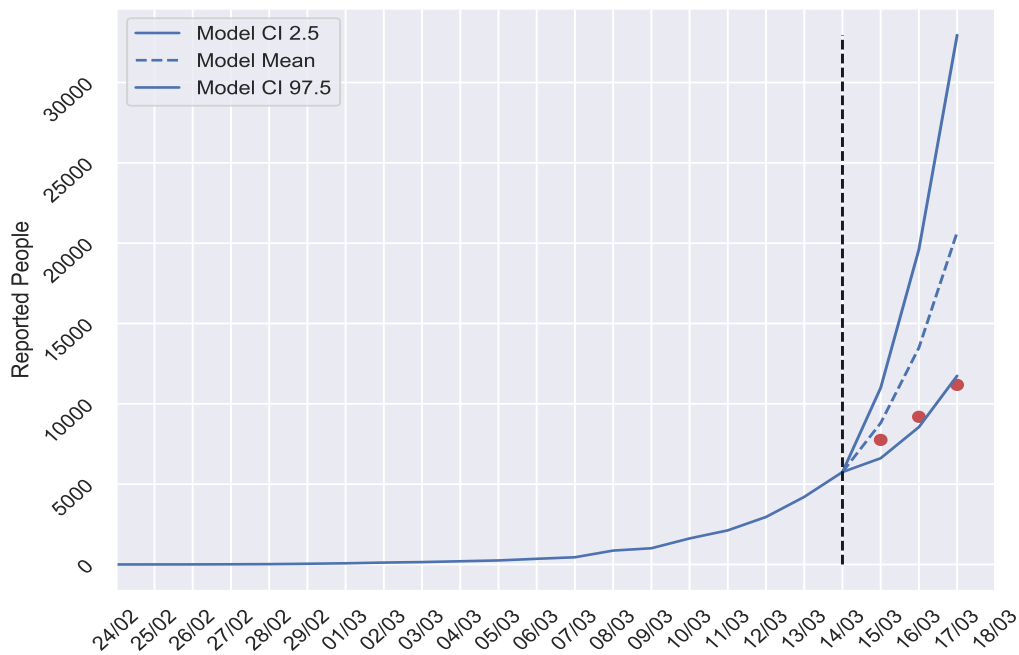
Figura 2: Predicción de reportados respecto al COVID-19 en ESPAÑA entre entre los días 14/03/2020 y 17/03/2020. Los puntos rojos corresponden a los datos publicados posteriormente a la realización de esta predicción. IMPORTANTE LEER APARTADO ACTUALIZACIÓN INFORME.
